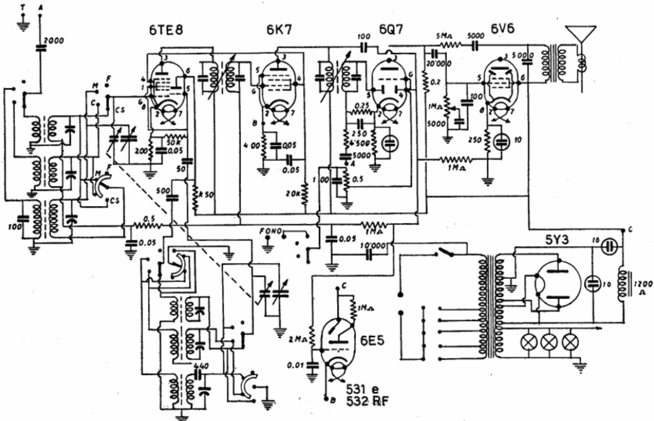
ZENIT RADIO - Modd. Z 530, Z 531 e Z 532 - Medie e due corte. Media frequenza 465 kc. Potenza d'uscita 4 watt.
